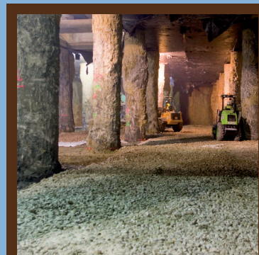
Depósito de Aguas de Tormenta Cuenca Centro Gijón
